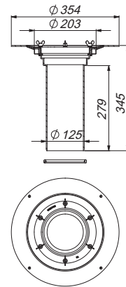
Aufstockelement 630 Schraubflansch
