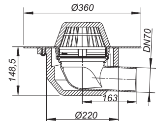
Dachablauf 64 PVC
