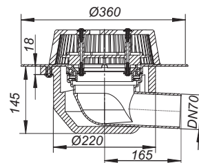
Aussparungsmaß: 240 x 320 mm
