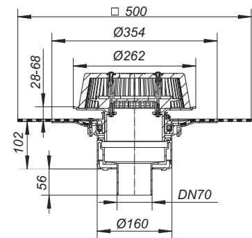
Notablauf SuperDrain 62 DallBit
