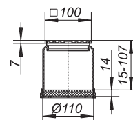
Aufsatz EC 10
