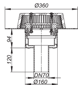
Aussparungsmaß: 170 x 320 mm Kernbohrungsmaß: d: 170 mm
