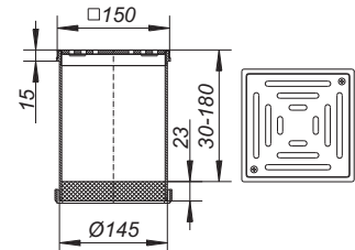
Terrassen-Aufsatz SES 15
