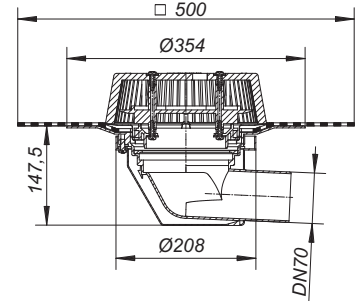
Aussparungsmaß: 265 x 320 mm
