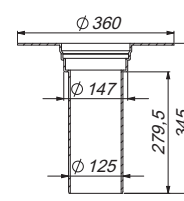
Aufstockelement 630 FPO-PE
