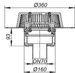
Aussparungsmaß: 170 x 320 mm Kernbohrungsmaß: d: 170 mm
