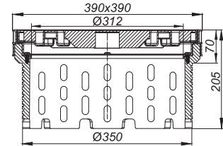
Drainage-Aufsatz 390 K
