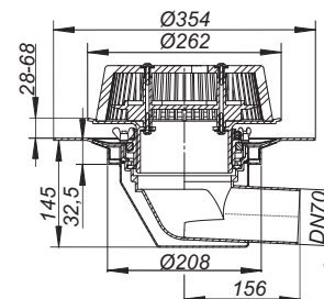
Aussparungsmaß: 265 x 320 mm
