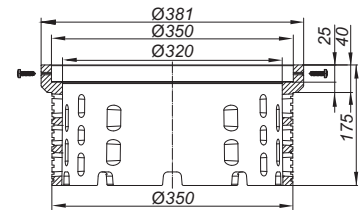
Drainage-Aufsatzverlängerung 390
