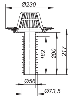
Sanierungs-Dachablauf 84 Schraubflansch
