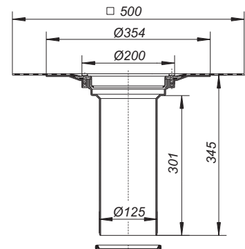
Aufstockelement 630 DallBit
