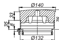
Notentwässerungseinheit 83/84
