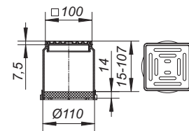
Aufsatz E 10
