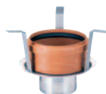
Brandschutzelement 1 für Betondach Nennweite Art.-Nr. Preis € DN 70 515018 230,40
