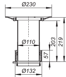
Aufstockelement 85
