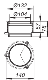
Einsteckmuffe 85
