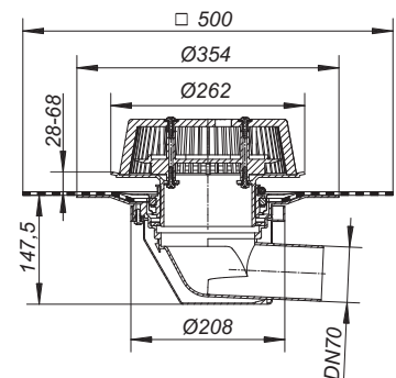
Notablauf SuperDrain 64 DallBit
