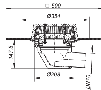
Dachablauf SuperDrain 64 DallBit
