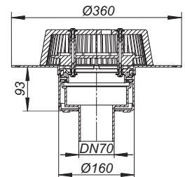
Dachablauf SuperDrain 62 PVC
