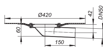
Balkonablaufgehäuse 83 DallBit
