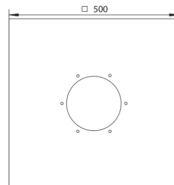
Anschluss-Manschette 65, PVC
