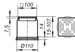
Aufsatz E 10
