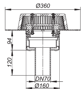
Dachablauf SuperDrain 62 FPO-PP
