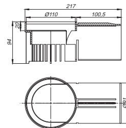
Entwässerungselement für Attikaabläufe
