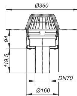
Dachablauf 62 FPO-PP
