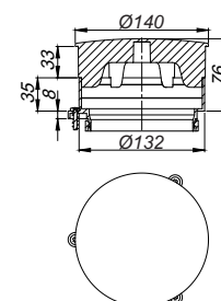
Notentwässerungseinheit 83/84
