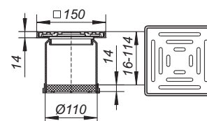
Aufsatz KE 10
