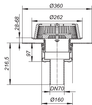
Notablauf SuperDrain 62 FPO-PP
