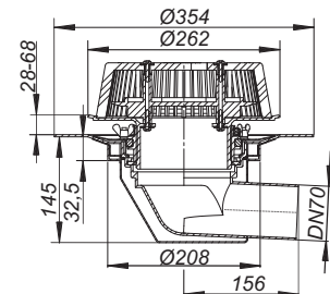
Notablauf SuperDrain 64 Schraubflansch
