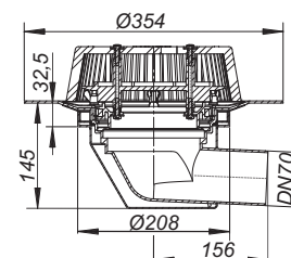
Dachablauf SuperDrain 64 Schraubflansch
