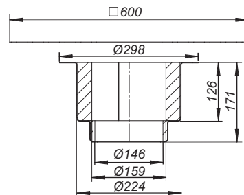
Brandschutzelement 9 Stahltrapez
