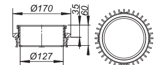
Einlafelement Umkehrdach
