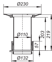
Aufstockelement 85
