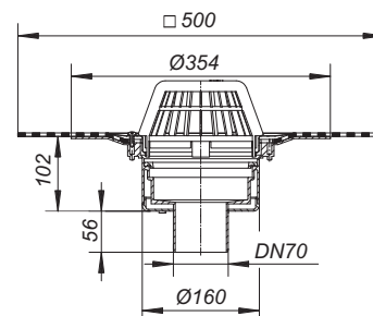
Dachablauf 62 DallBit
