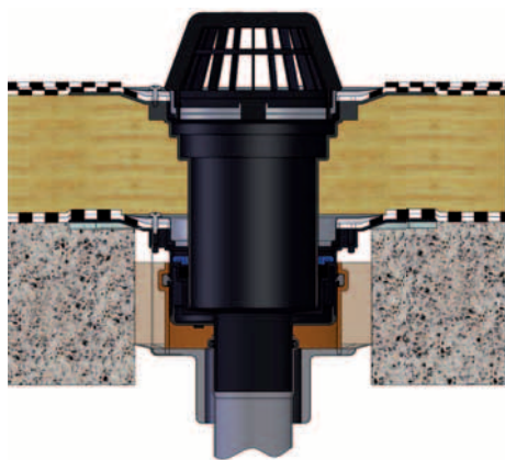
Brandschutzelement 1 mit Dachablauf 62 und Aufstockelement 630
