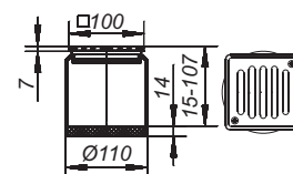
Aufsatz ECS 10
