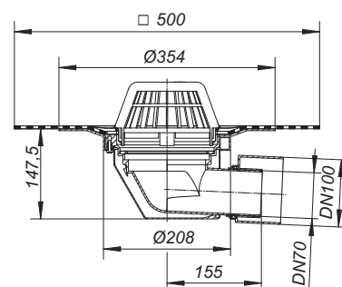
Dachablauf 64 DallBit
