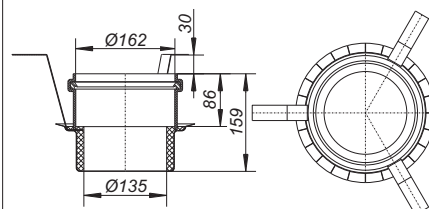
Brandschutz-Rohbauelement 5
