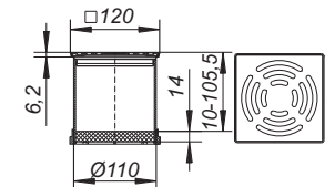
Aufsatz E 12
