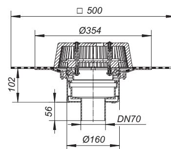
Dachablauf SuperDrain 62 DallBit
