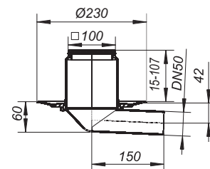
Balkonablauf 83 E
