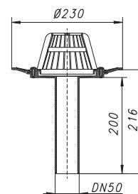
Aussparungsmaß: 180 x 250 mm
