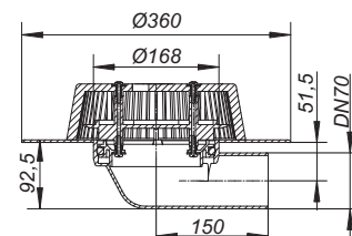
Power-Dachablauf 86.0 PVC
