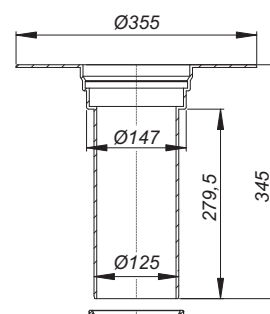
Aufstockelement 630 PVC
