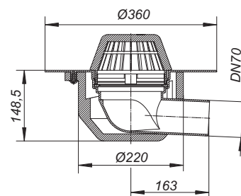
Dachablauf 64 FPO-PP
