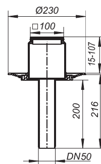
Balkonablauf 84 E
