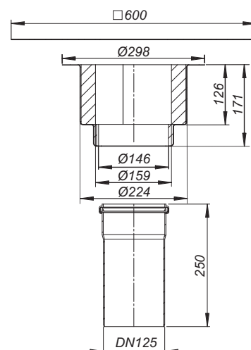
Brandschutzelement 10 Stahltrapez
