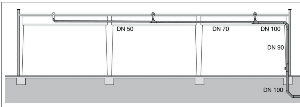
Druckströmungsentwässerungs-System (DSS)
