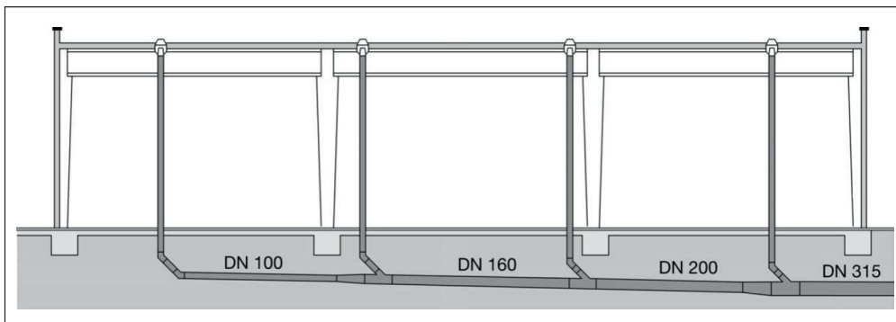
Freispiegelentwässerungs-System (FSE)
