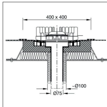
PE Dachablauf DSS - Kaldach Massivbau und Leichtbau
