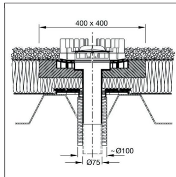
PE Dachablauf DSS - Warmdach Massivbau und Leichtbau
