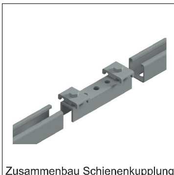
Zusammenbau Schienenkupplung
